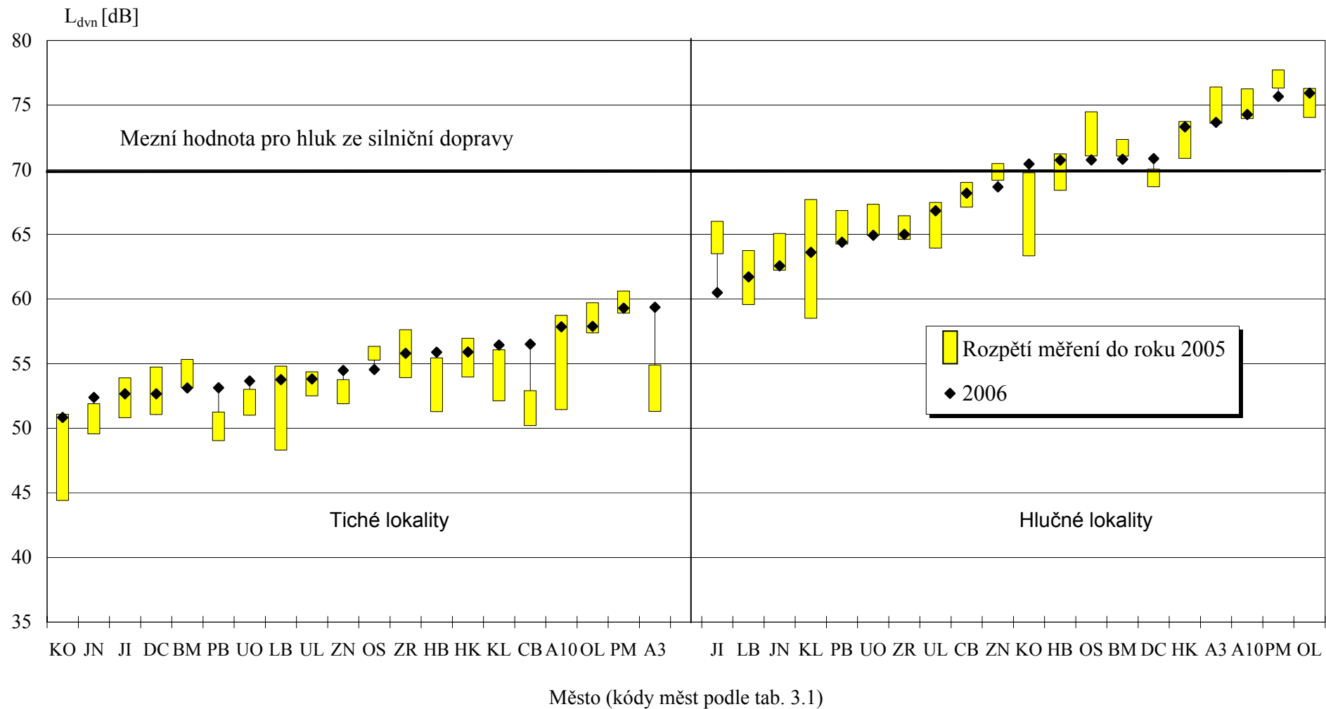
Obr. 4 Hlukový ukazatel pro den - večer - noc L_{dvn} (24 hodin)
